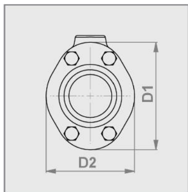
DN10 - DN50
