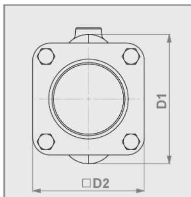
DN65 - DN100
